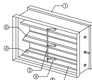
5) Stopper Strip
